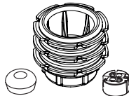
Verbindungssatz (513-0230) Befestigungsmutter mit 3 Silikon- scheiben für 1,5mm 2 Kabel
